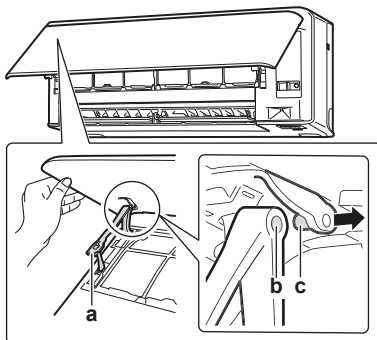
a Рычаг b Гнездо стержня c Шток
