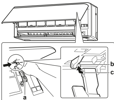
a Рычаг b Шток c Гнездо стержня
