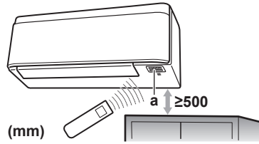
a Приемник сигнала
